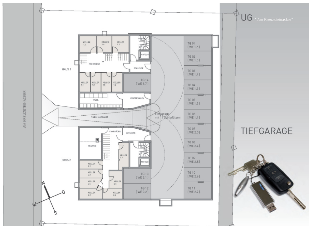
Untergeschoss TG
