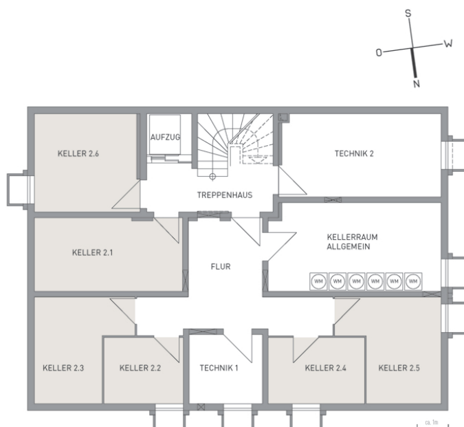
Haus 2 UG
